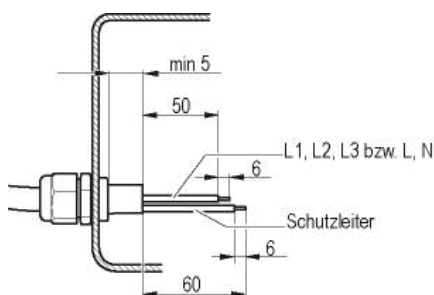
Abb. 1: Empfohlene Abmantellängen in mm (innerhalb Klemmkasten)
